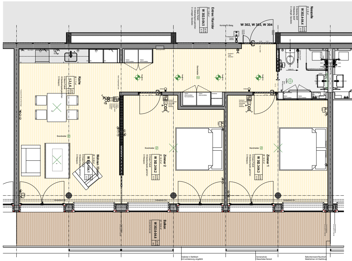
Grundriss Typ 3.1_3.5-Zi Wohnung
