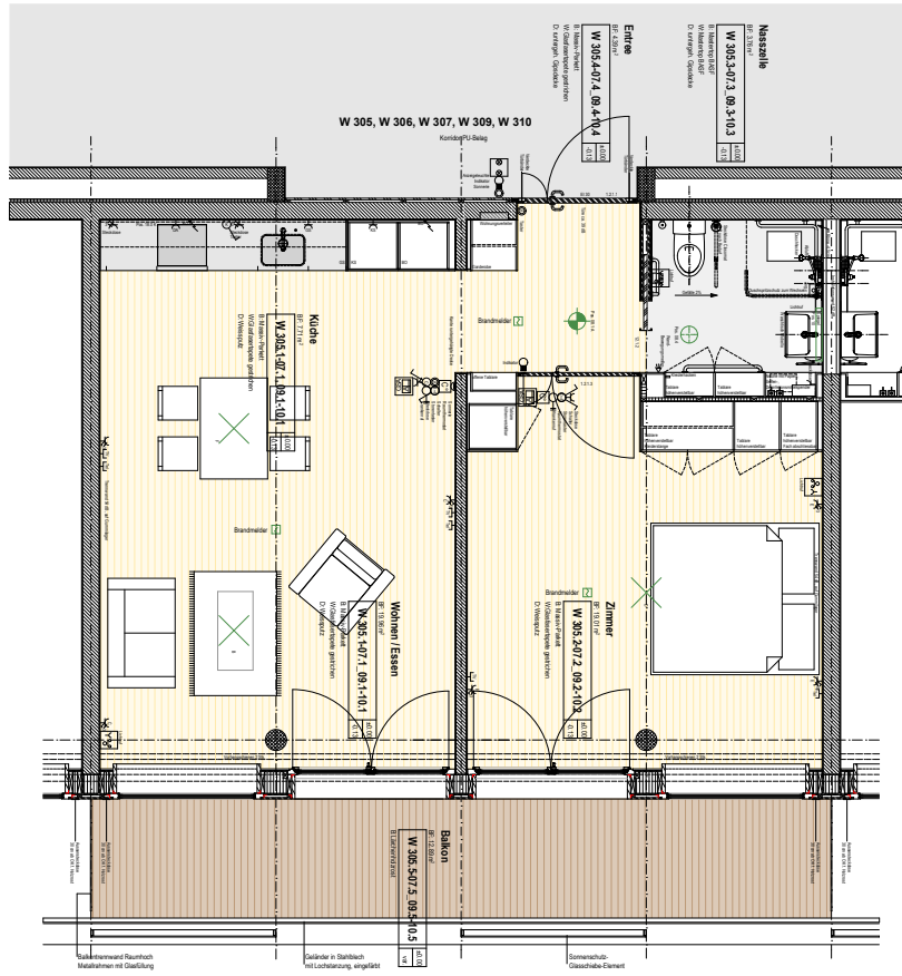
Grundriss Typ 2.1_2-Zi Wohnung
