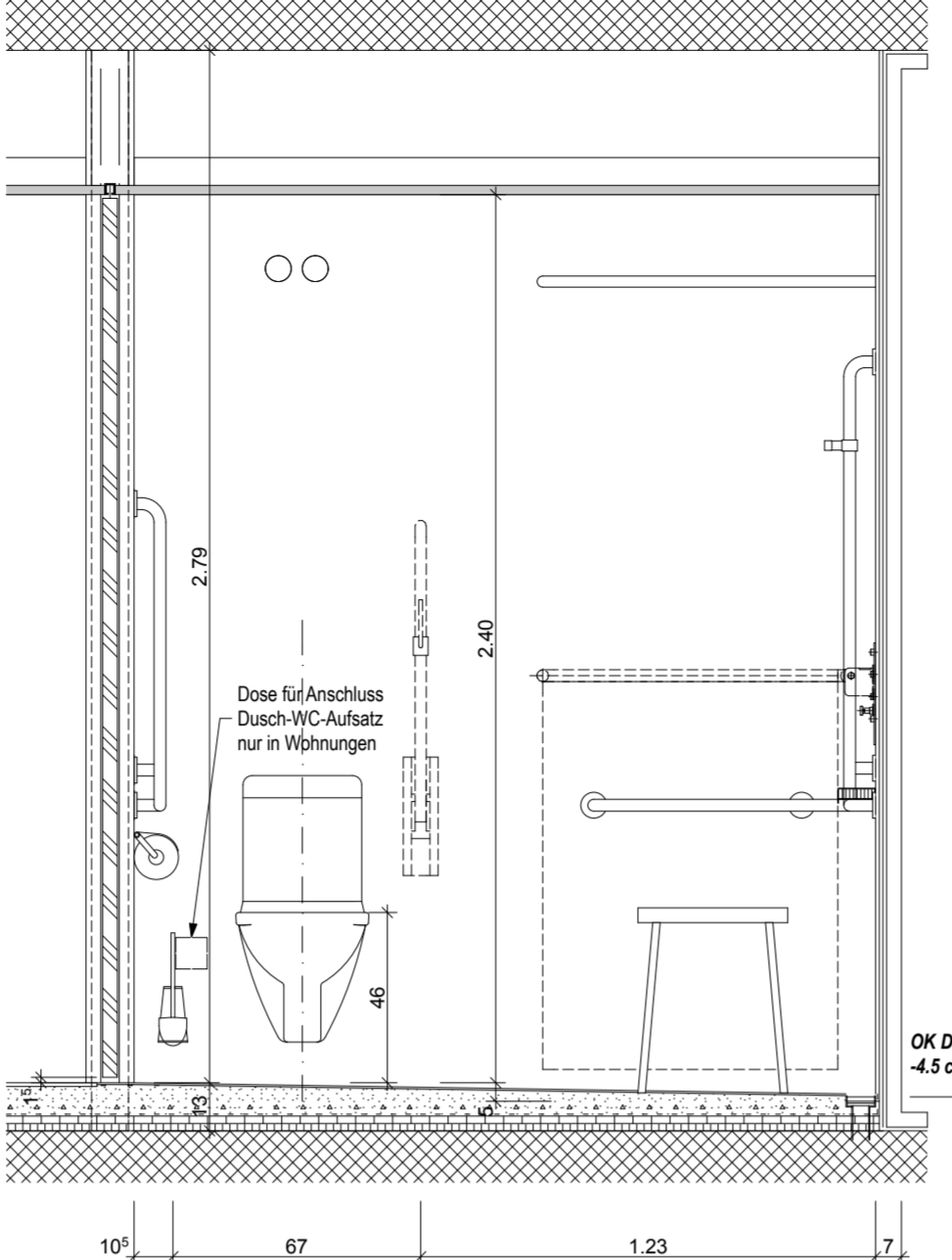
Schnitt / Ansicht B-B
