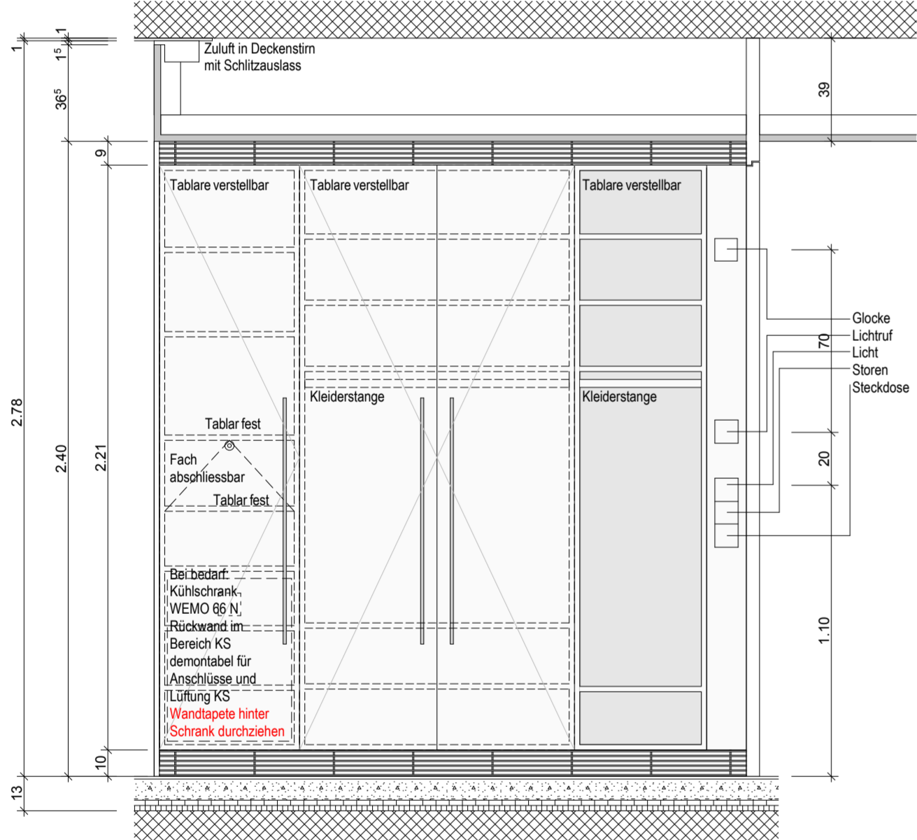
Ansicht Schrankfront Entree
