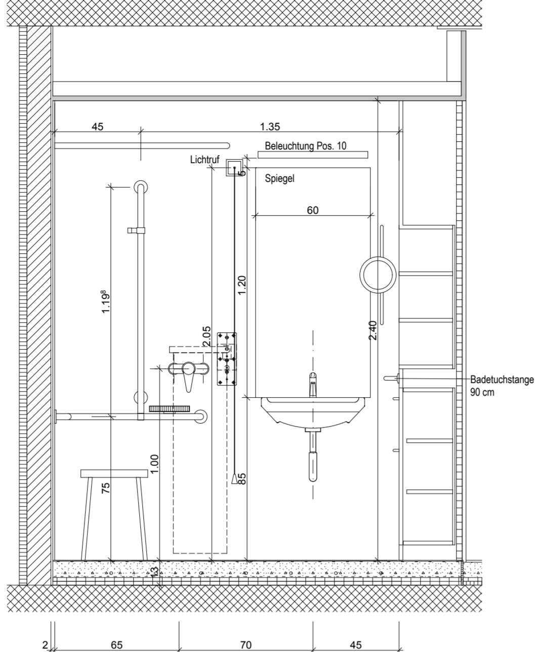
Schnitt / Ansicht A-A
