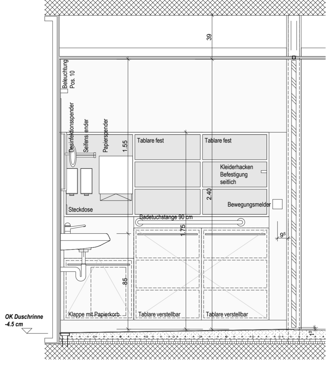
Schnitt / Ansicht D-D
