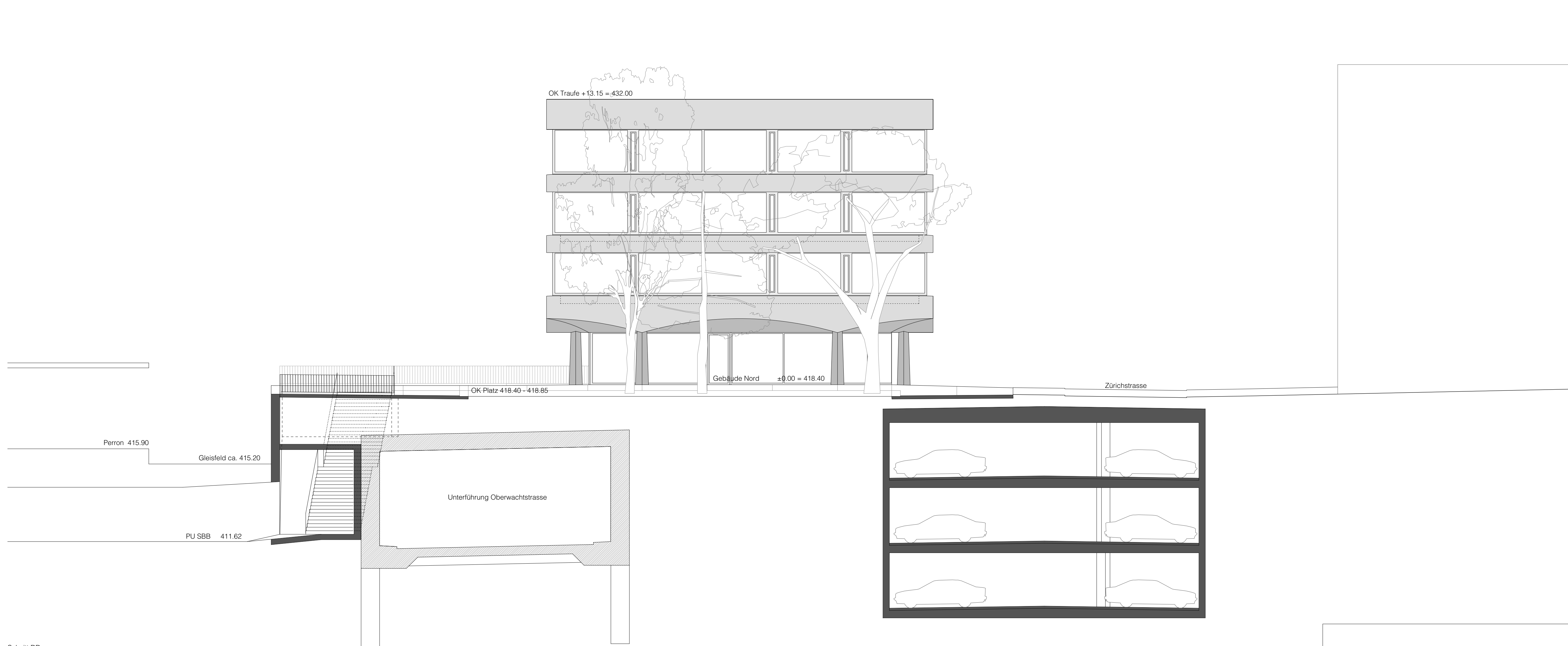
Schnitt DD
