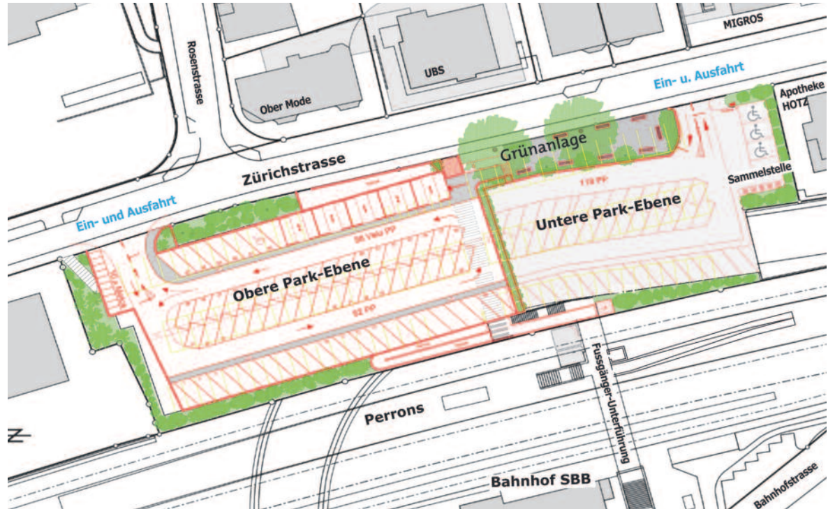
Grundriss des Alternativprojektes mit insgesamt 180 Parkplätzen.
