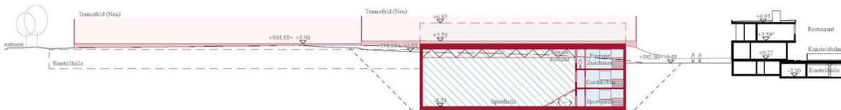
Querschnitt durch Sporthalle und KEK-Betriebsgebäude
